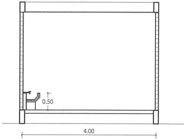
รูปตัด A - A มาตรฐาน 1 : 50
