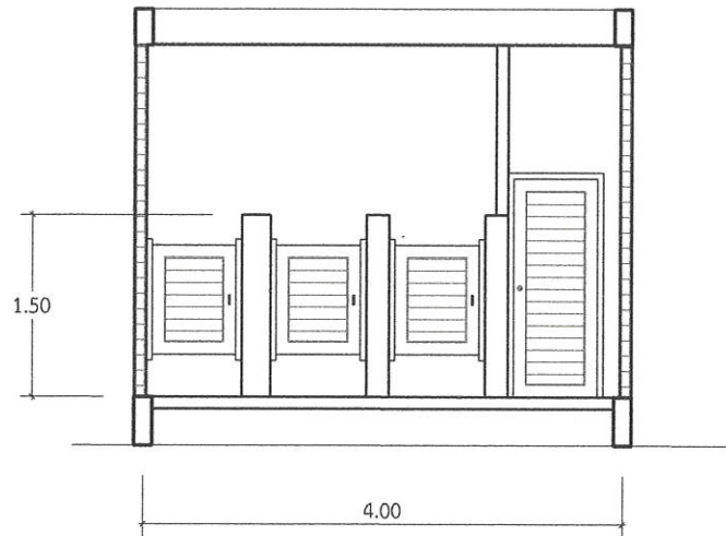
รูปตัด B - B มาตรฐาน 1 : 50
