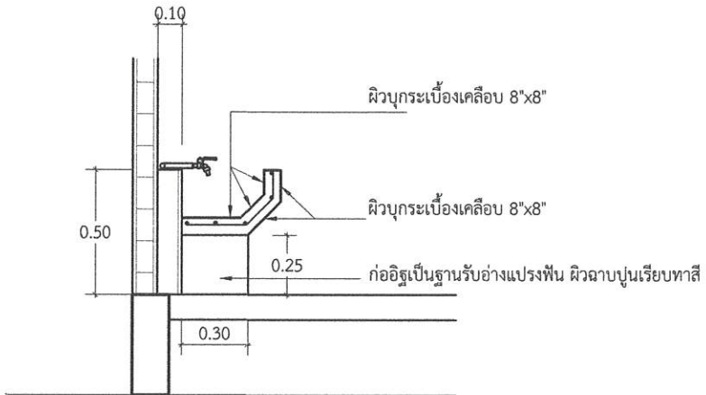
ขยายอ่างล้างหน้า มาตรฐาน 1 : 20
