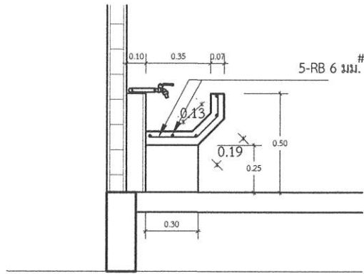
ขยายอ่างล้างหน้า มาตรฐาน 1 : 20
